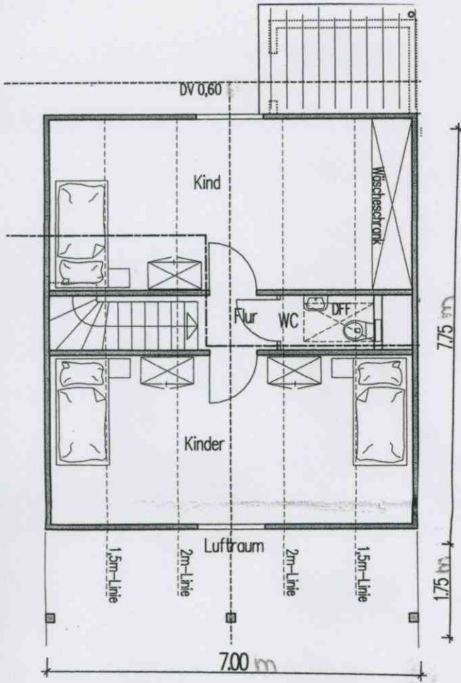
GRUNDRISS DACHGESCHOSS
