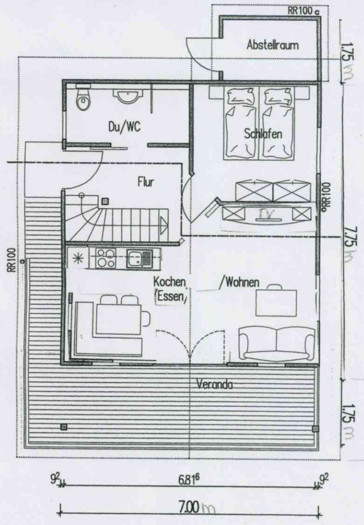
GRUNDRISS ERDGESCHOSS
